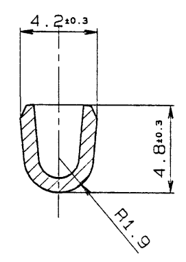
SEC. A-A
