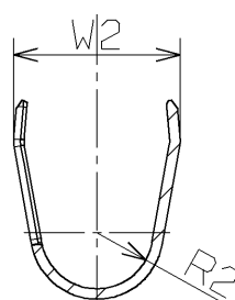
SEC. B-B(L SIZE)
