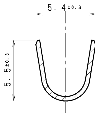
SEC. A-A
