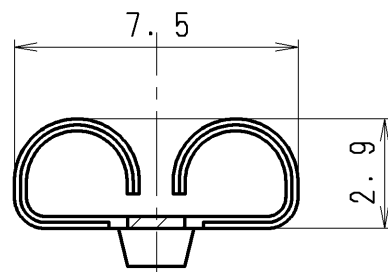
SEC. A-A
