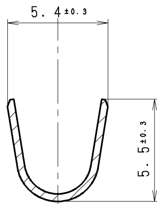
SEC. A-A
