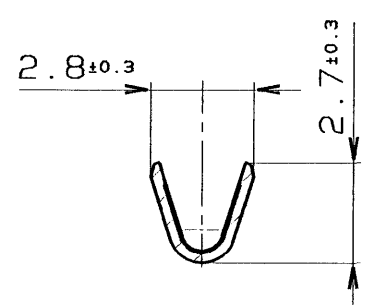
SEC. A-A
