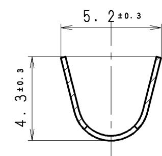
SEC. A-A
